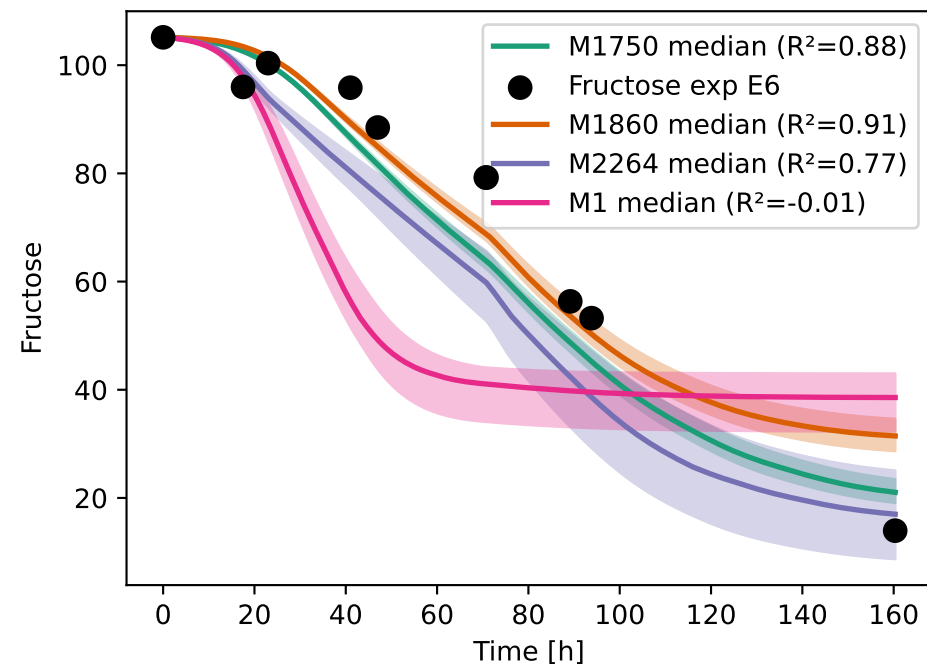
Fructose
